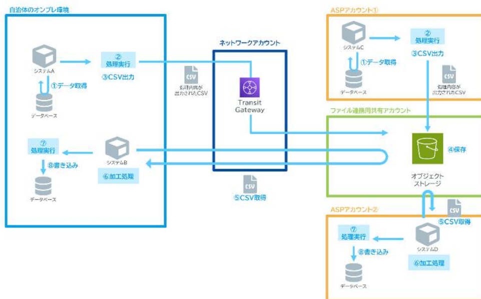
図 ファイル連携の構成イメージ
